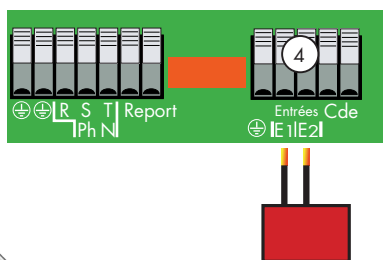
Compteur à impulsion
