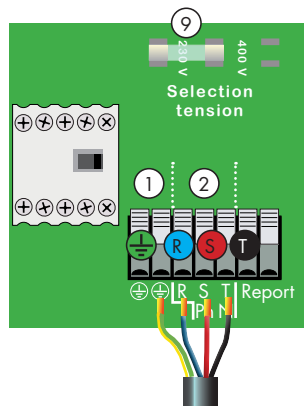
Alimentation 400 V
