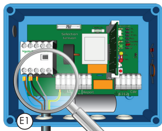
Pompe monophasée 230 V
